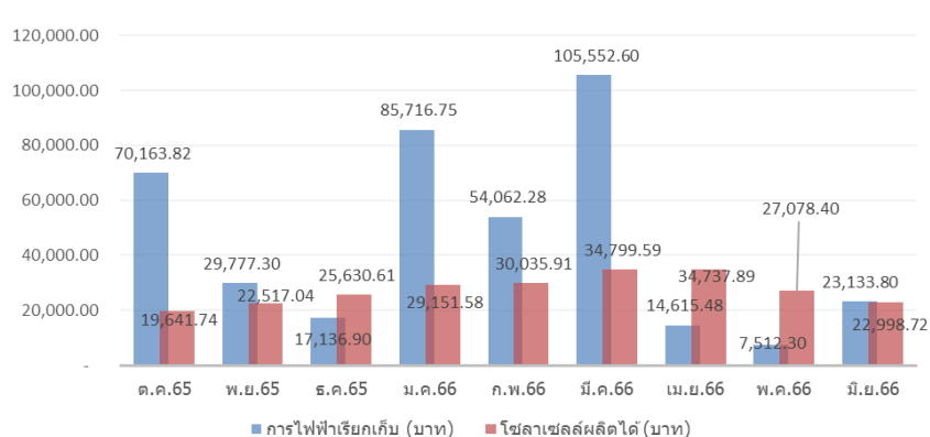
กราฟแสดงการใช้ไฟฟ้า และการผลิตไฟฟ้าจากโซลาเซลล์ อาคารกิจกรรมและนันทนาการ
